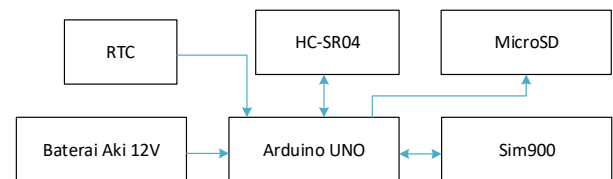
Gbr 2. Konfigurasi Alat
